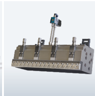
XD-25XW 400mm
